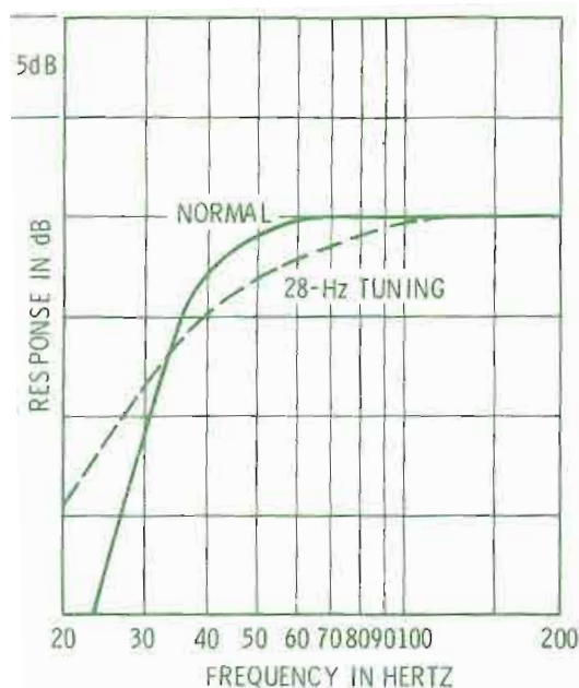
Fig. 5 28 Hz Tuning
